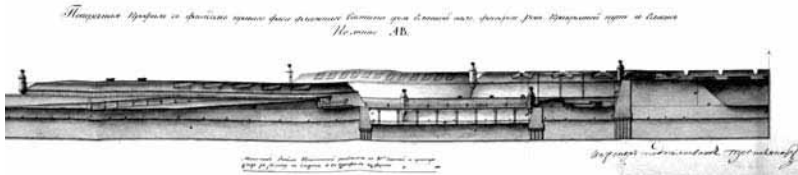
Ил. 5. Поперечный профиль (разрез) правого фаса Флажного бастиона через главный вал, фоссебрею, ров и гласис. Показаны артиллерийские позиции на главном валу и гласисе. Фрагмент чертежа. 1810 г. РГВИА
