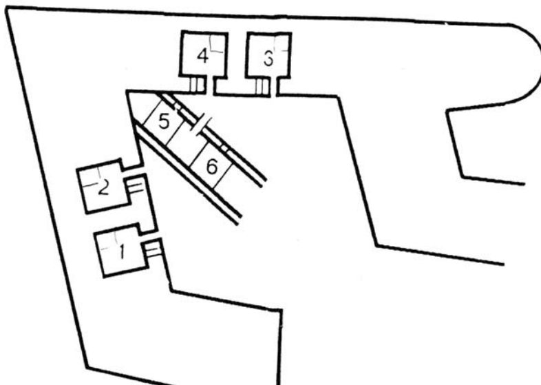
Ил. 2. Расположение и нумерация камер в Зотовом бастионе. Реконструкция М. В. Вершевской
