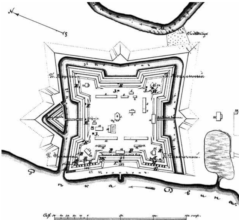
Ил. 6. Фрагмент чертежа Новодвинской крепости 1853 г. РГВИА
